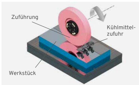
Horizontale Spindel, Pendeltisch
