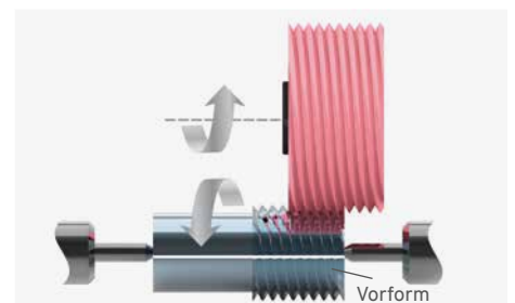
Gewindeschleifen im Einstechverfahren
