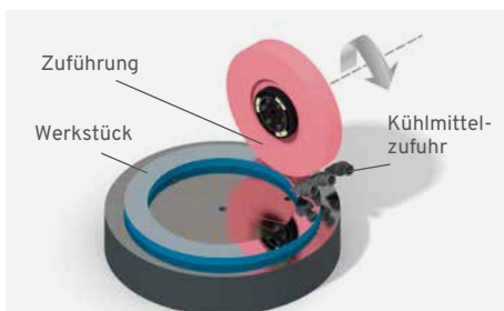
Horizontale Spindel, Rundtisch
