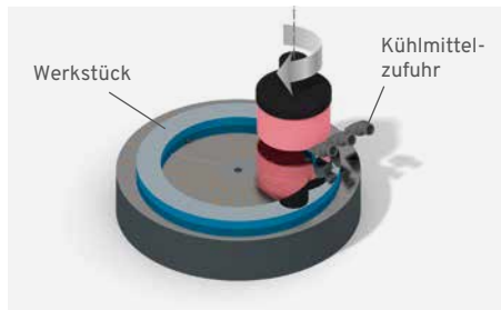
Vertikale Spindel, Rundtisch
