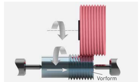
Schleifen von Quergewinden
