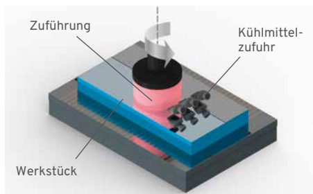
Vertikale Spindel, Pendeltisch
